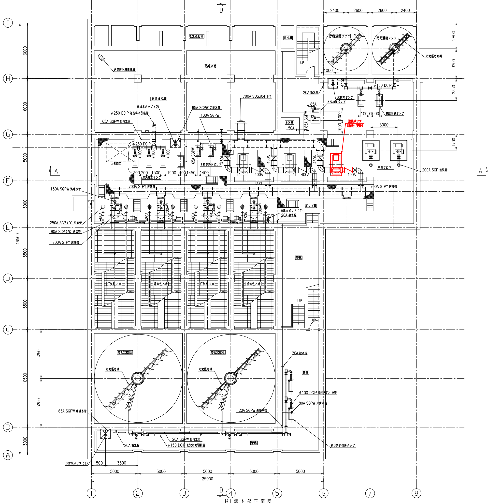
B1階下部平面図
